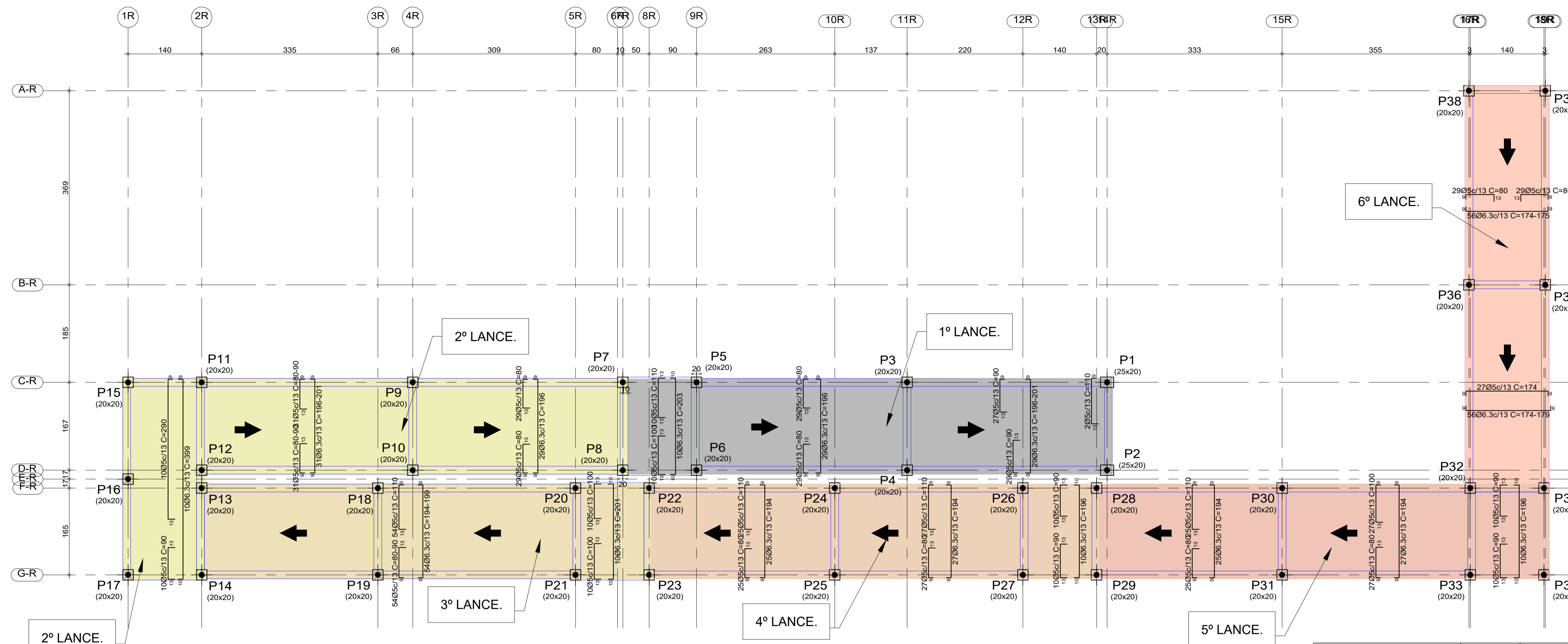
ARMADURA DA LAJE - RAMPA INTERNA (NÍVEL INFERIOR/TERREO - COTA: 361,50 À 365,00)
