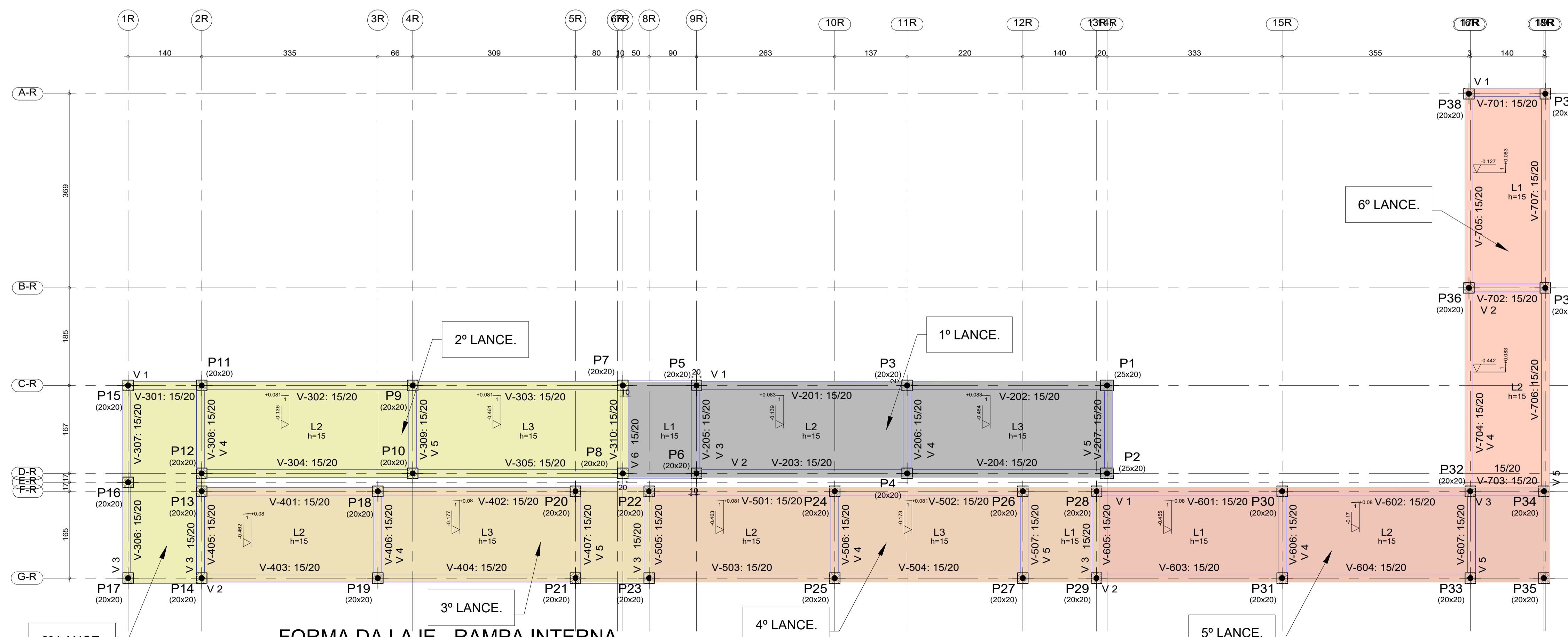
FORMA DA LAJE - RAMPA INTERNA (NÍVEL INFERIOR/TERREO - COTA: 361,50 À 365,00)
