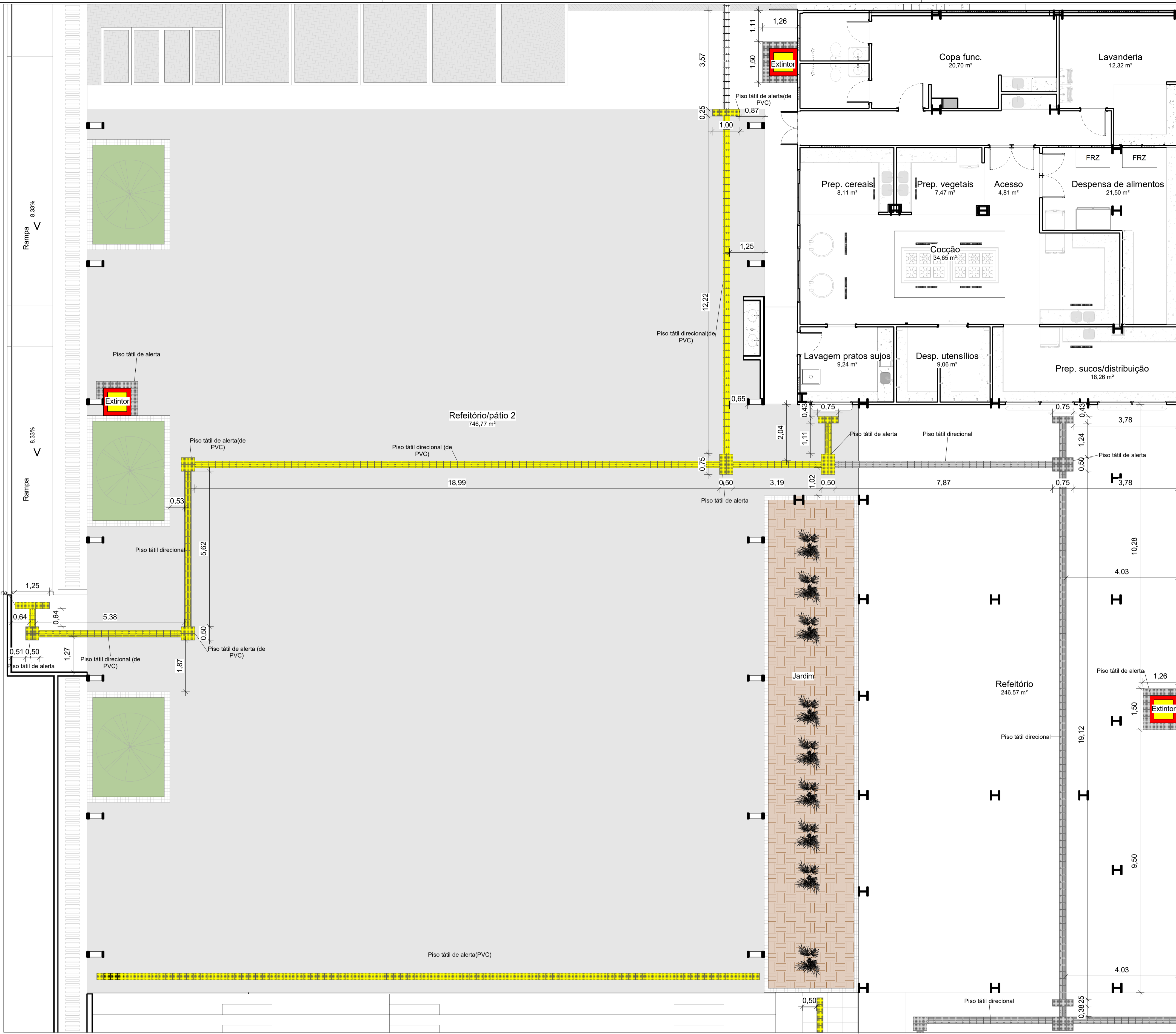
1 TATIL-PB-recorte Cozinha/acesso Escala: 1 : 75
