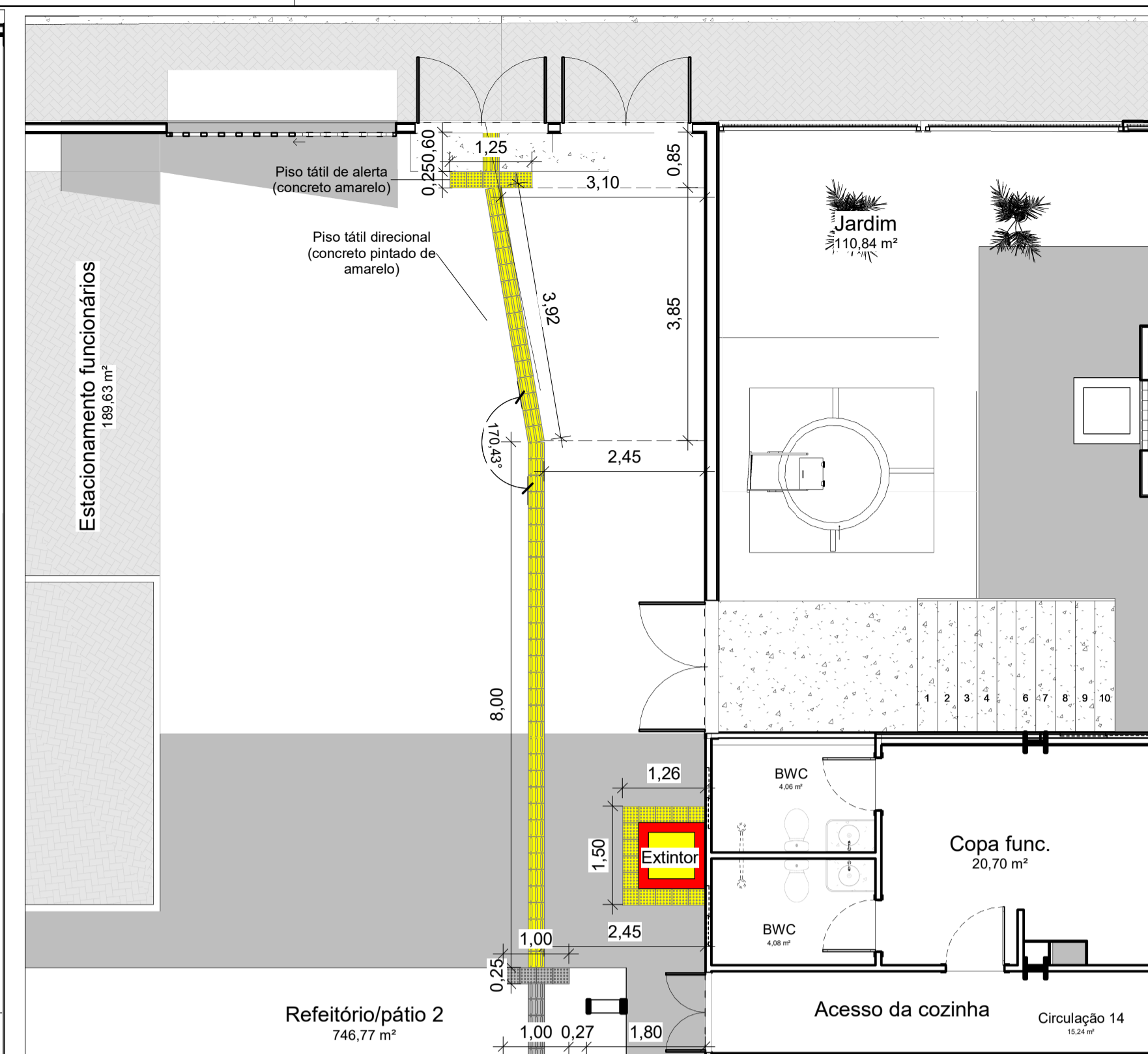
2 TATIL-PB-recorte acesso do portao da cozinha Escala: 1 : 75
