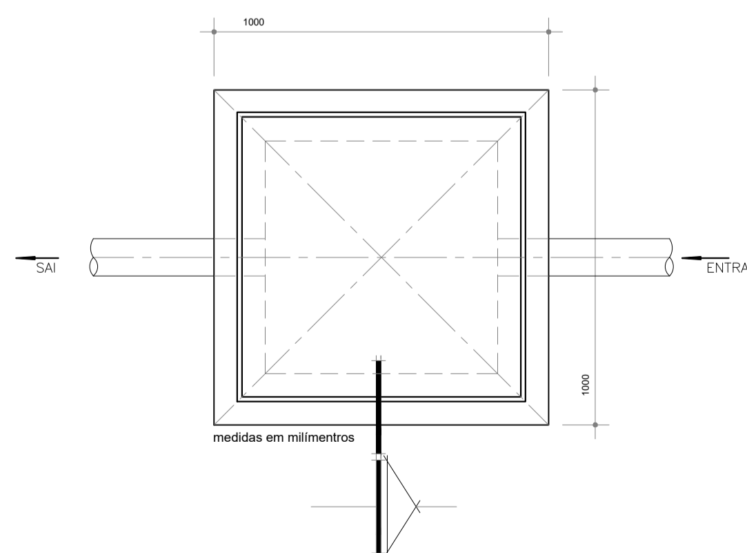
VISTA SUPERIOR CAIXA DE INSPEÇÃO SEM ESCALA
