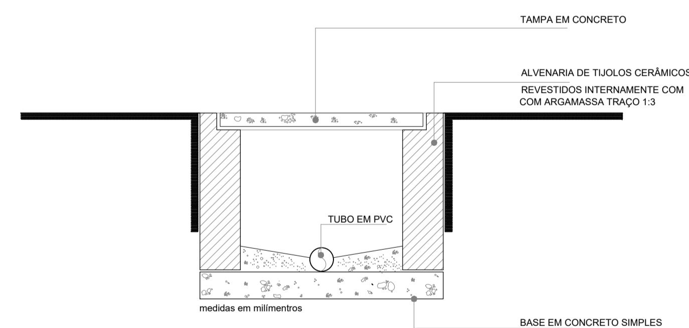
CORTE CAIXA DE INSPEÇÃO SEM ESCALA
