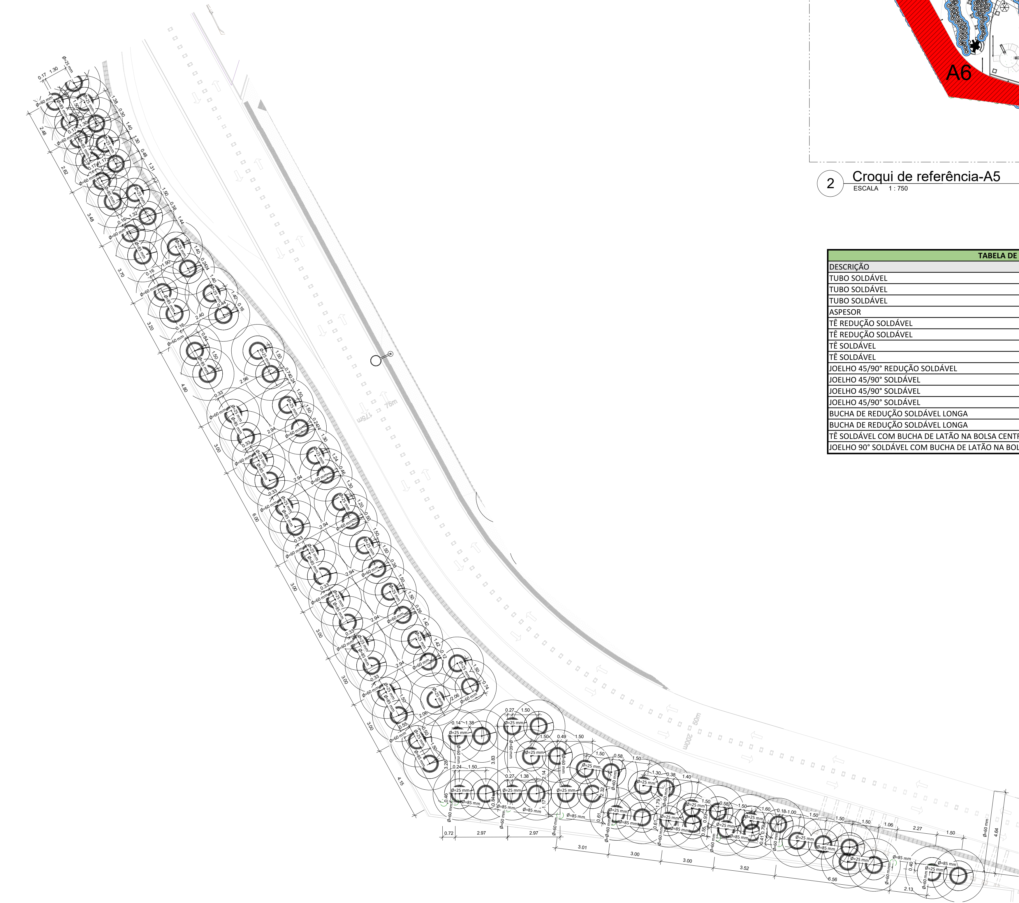
1 Planta de locação das mudas - A5 ESCALA 1:125
