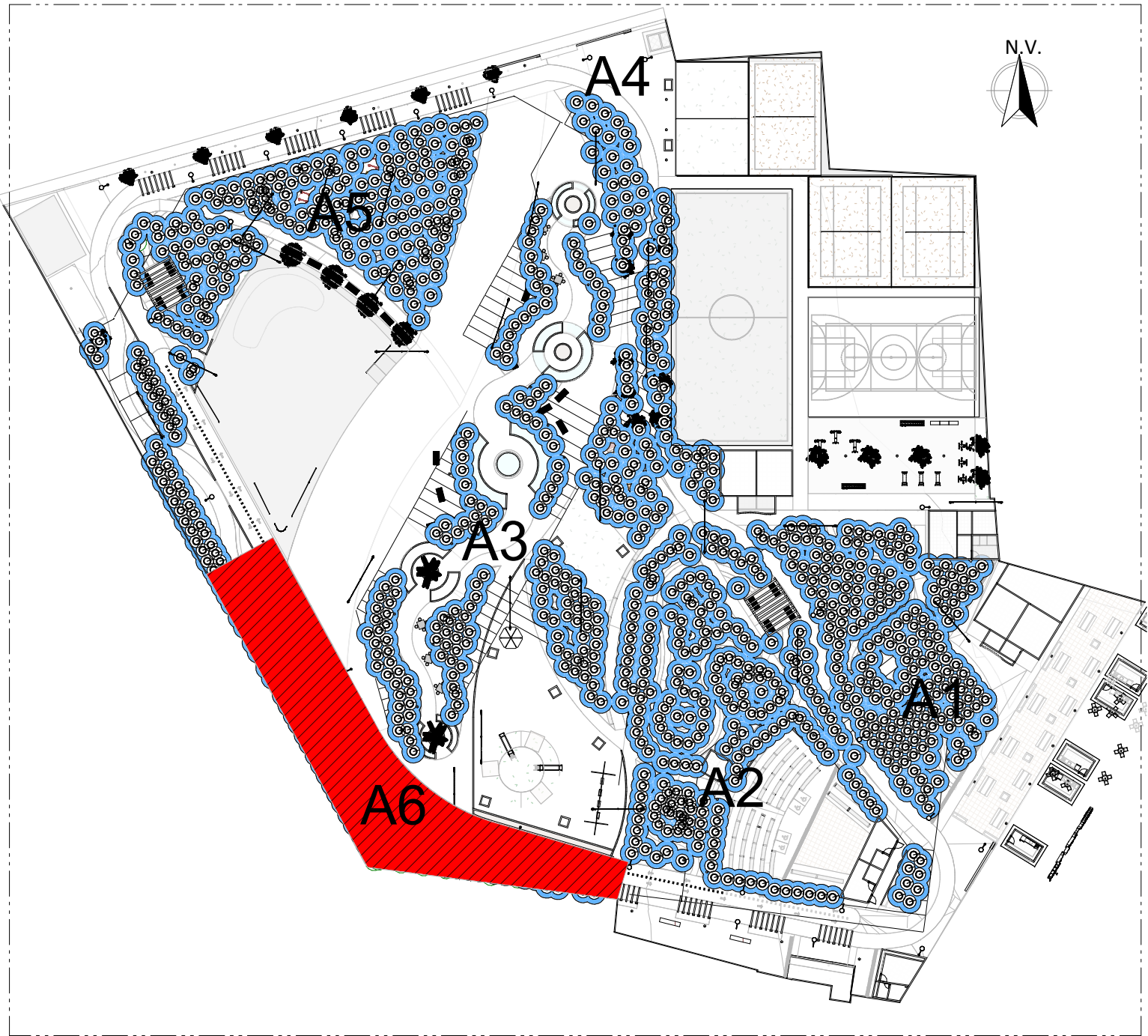
2 Croqui de referência-A5 ESCALA 1:750
