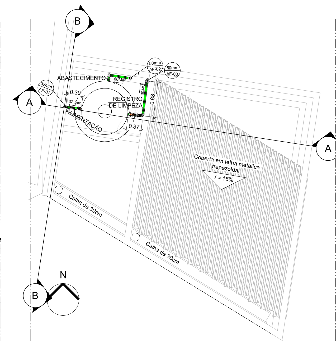
2 CENTRAL DE SEGURANÇA - PLANTA DE COBERTA ESCALA 1:50
