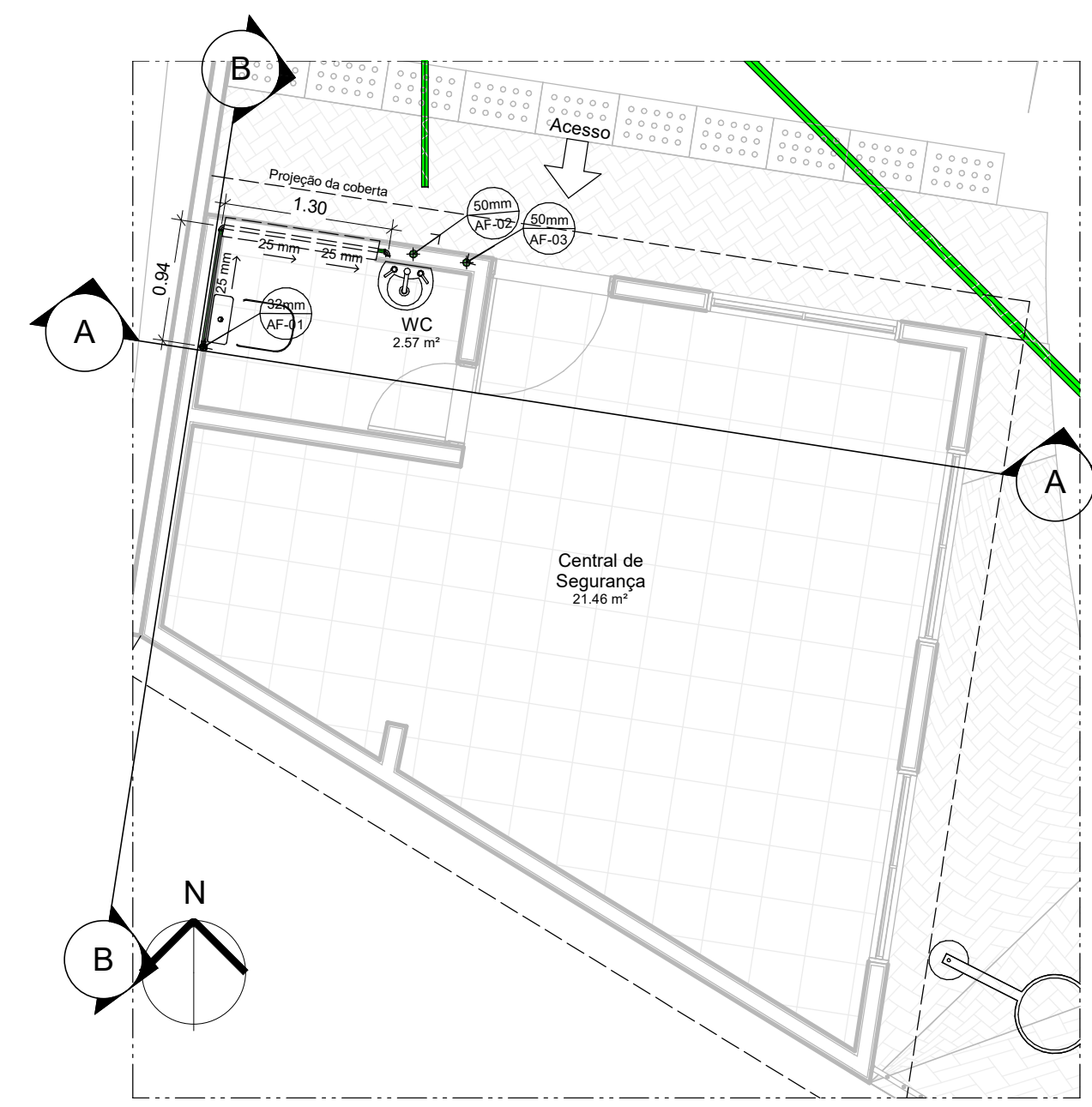
3 CENTRAL DE SEGURANÇA - PLANTA BAIXA ESCALA 1:50
