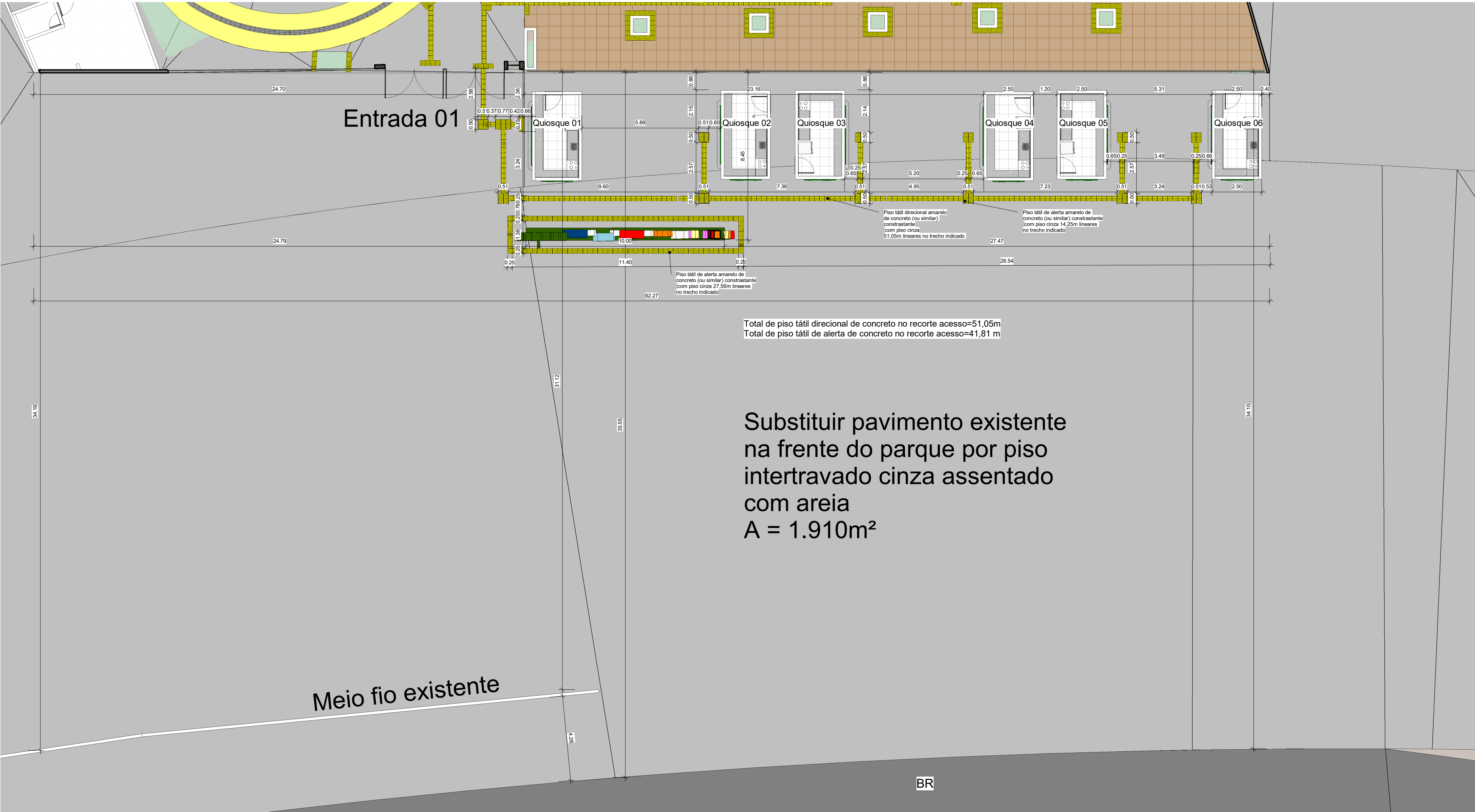
1 Planta de pag. de piso-Acesso Entrada 01
