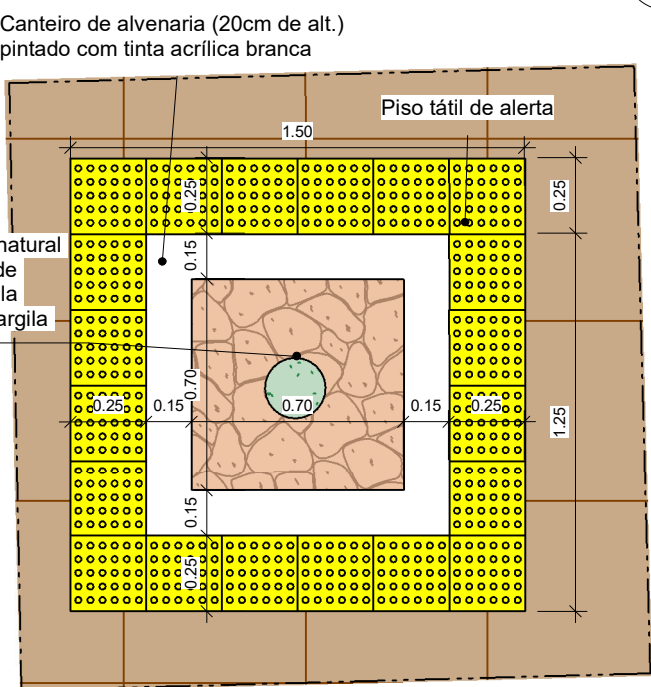
4 Det. 01-Alegrete-Picnic ESCALA 1:25
