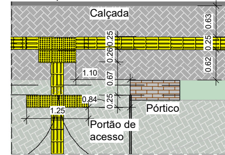
4 Det.06 - Piso tátil entrada 02 ESCALA 1:75
