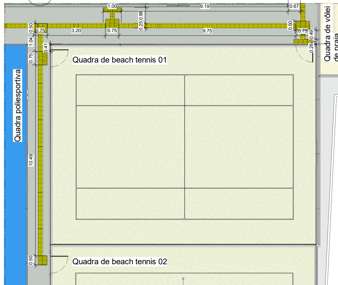
5 Planta de localização do piso tátil-Acesso as quadras de beach tennis ESCALA 1 : 125
