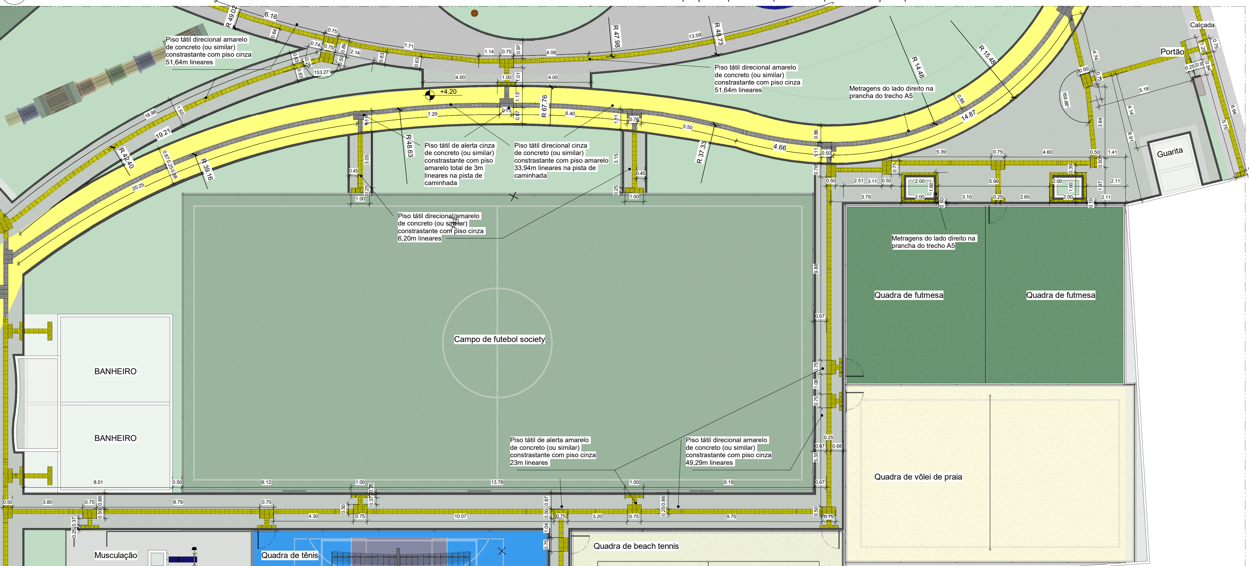
1 Planta de localização do piso tátil A4 ESCALA 1 : 125
