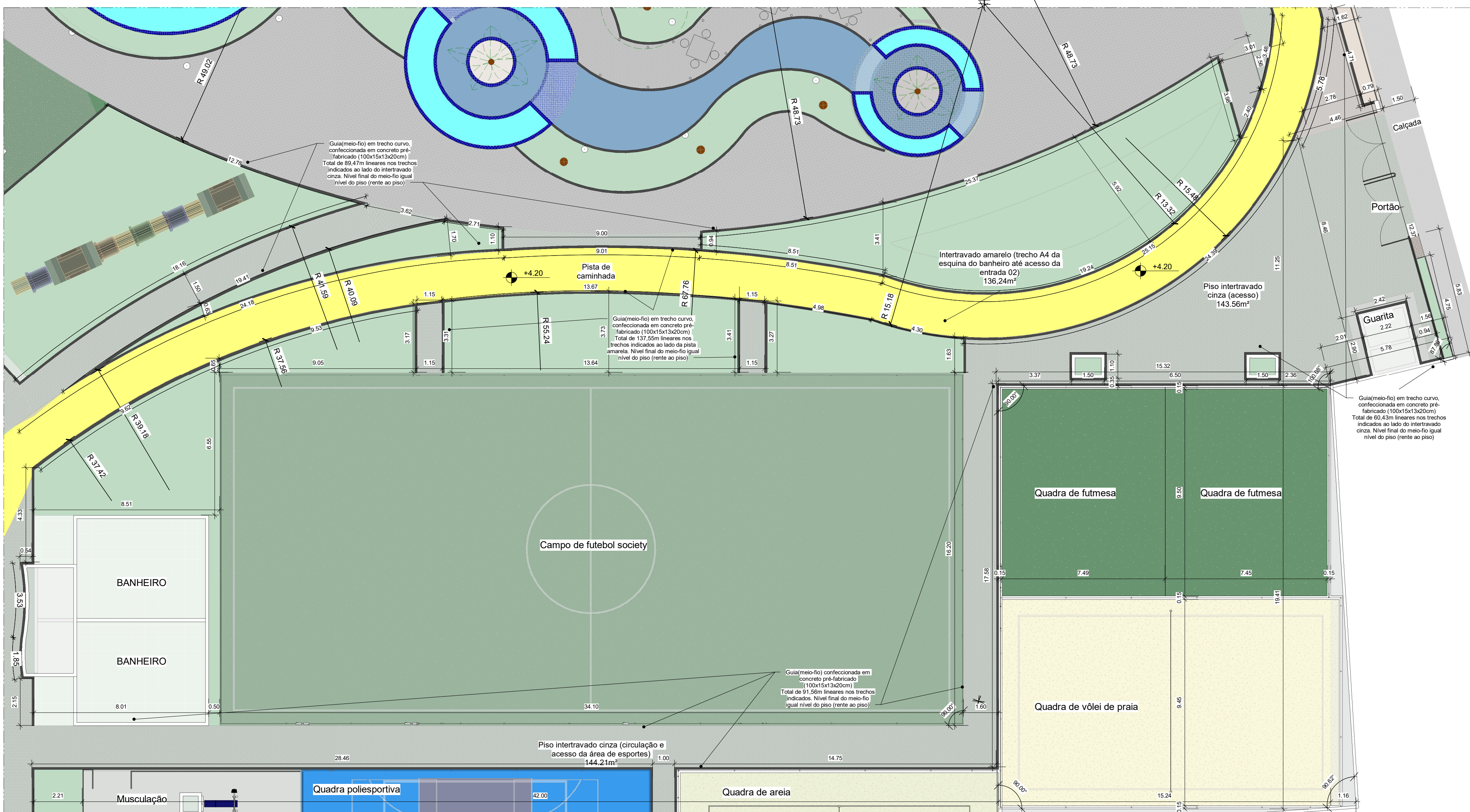
2 Planta de localização do piso tátil A4 ESCALA 1 : 125
