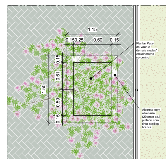
4 Det.06-Alegretes-A4 ESCALA 1:50
